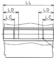
Rスナップリング溝 R snap ring groove (両側) (Both)
